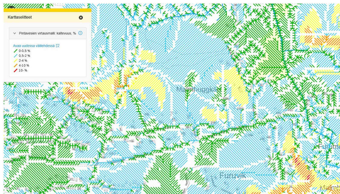
Bild 6. Lutning (%) enligt flödesmodellen för ytvatten. Källa: Paikkatietoikkuna, 2025. Material: Finlands skogscentral, 2018.
