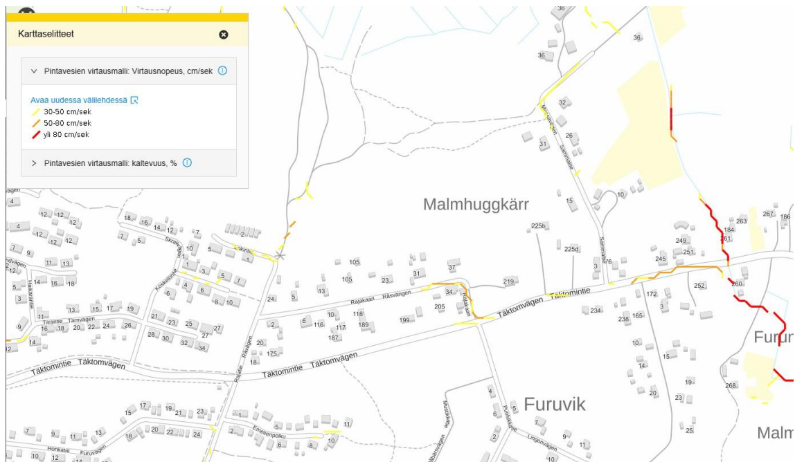
Bild 7. Flödes hastighet (cm/s) enligt flödesmodellen för ytvatten. Källa: Paikkatietoikkuna, 2025. Material: Finlands skogscentral, 2018.
